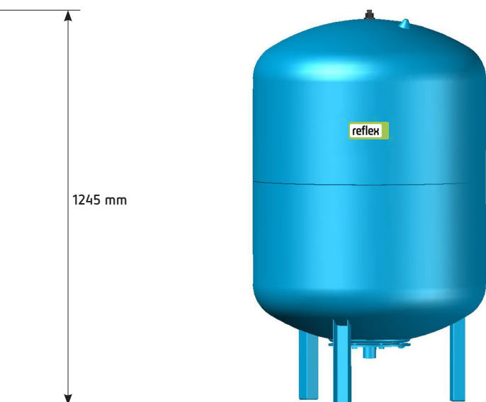
Reflex DE 400 litri / 10 bar
