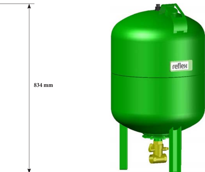
Reflex DT 100 litri/10 bar
