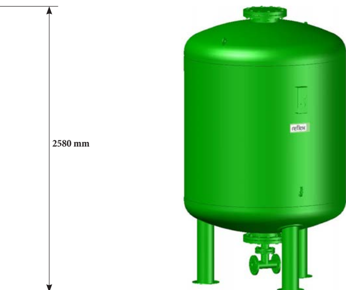
Reflex DT 3000 litri/16 bar
