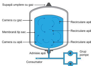
Schemă funcțională vas de expansiune Reflex DD și DT, cu membrană tip sac și cu recirculare (imagine cu caracter ilustrativ)
