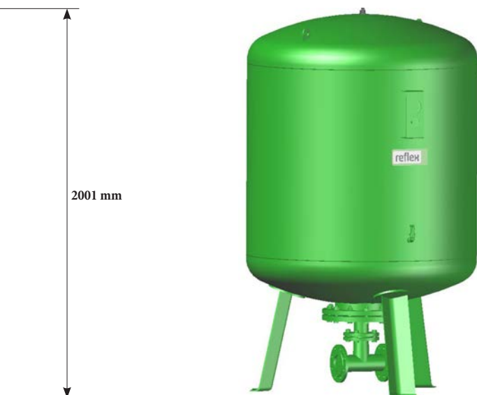
Reflex DT 1500 litri/10 bar
