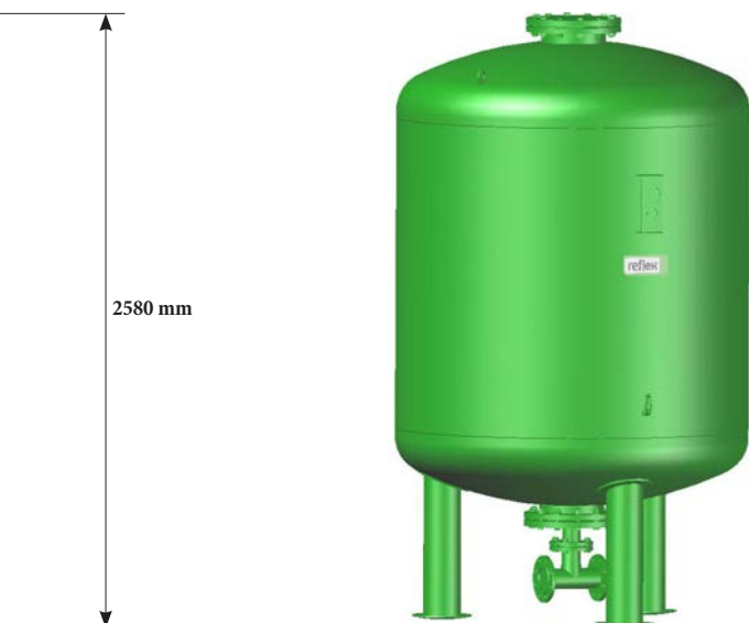
Reflex DT 3000 litri/16 bar
