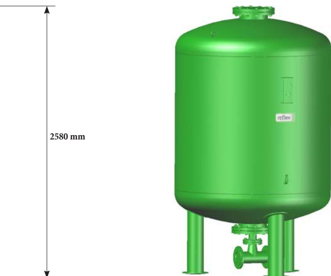
Reflex DT 3000 litri/16 bar
