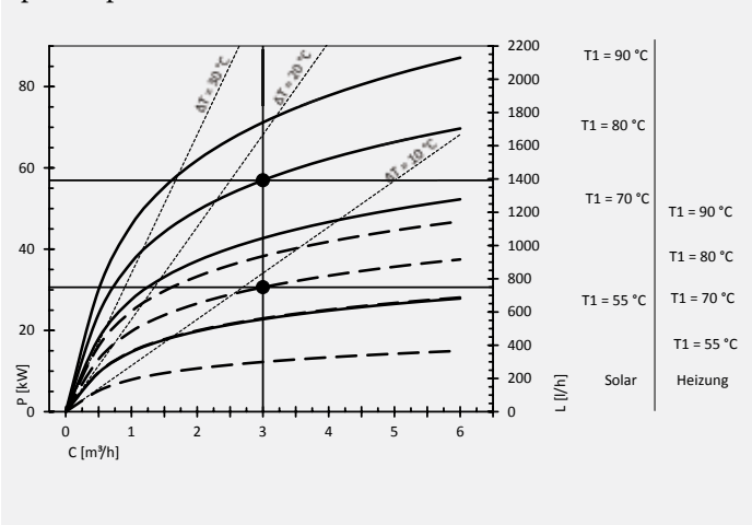
Diagrame de performanță Storatherm Aqua Solar 400/2 pt. temperatura de 45°C
