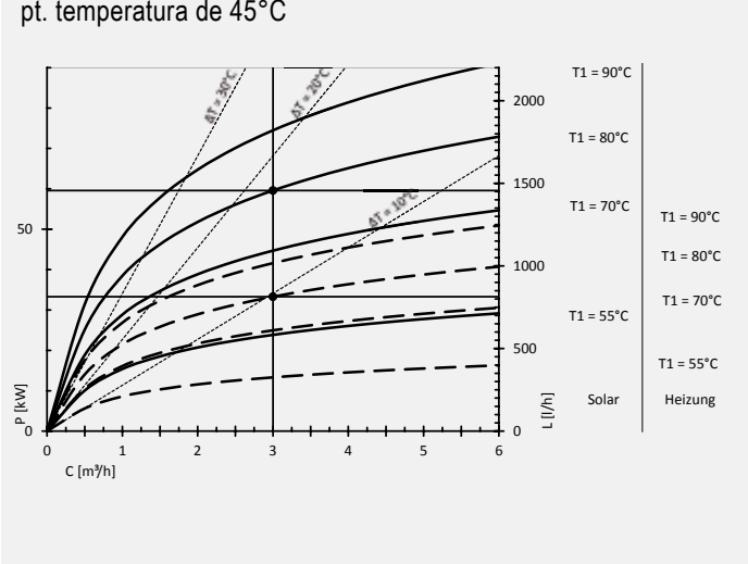
Diagrame de performanță Storatherm Aqua Solar 750/2
