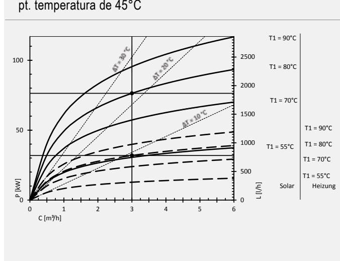
Diagrame de performanță Storatherm Aqua Solar 1000/2
