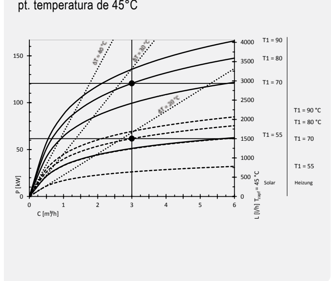
Diagrame de performanță Storatherm Aqua Solar 2000/2
