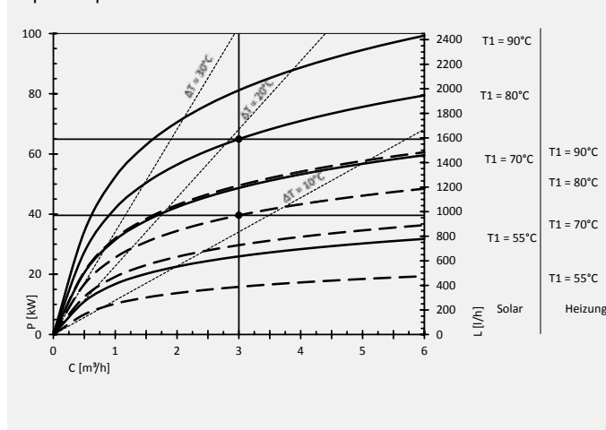
Diagrame de performanță Storatherm Aqua Solar 500/2 pt. temperatura de 45°C
