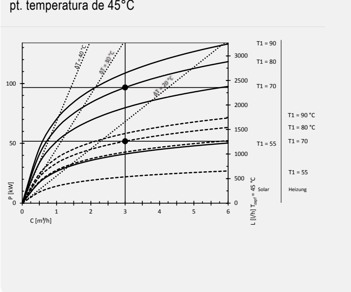
Diagrame de performanță Storatherm Aqua Solar 1500/2
