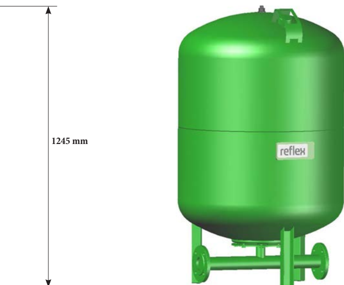
Reflex DT 400 litri/10 bar
