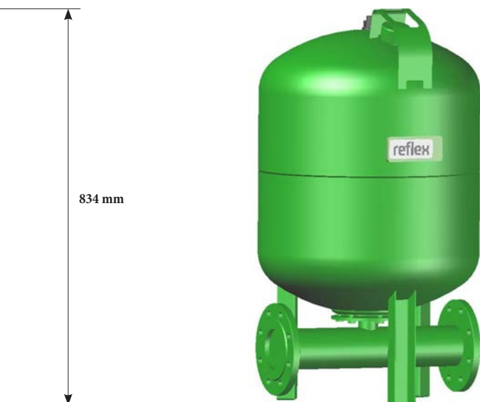
Reflex DT 100 litri/16 bar
