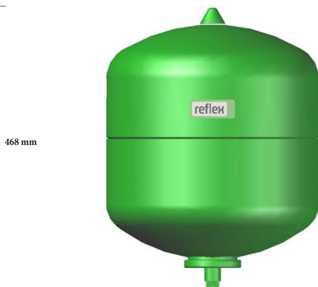
Reflex DD 33 litri/10 bar
