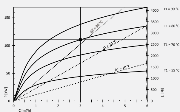
Diagrama de performanță Storatherm Aqua 1000/1 la o temperatură de 45°C
