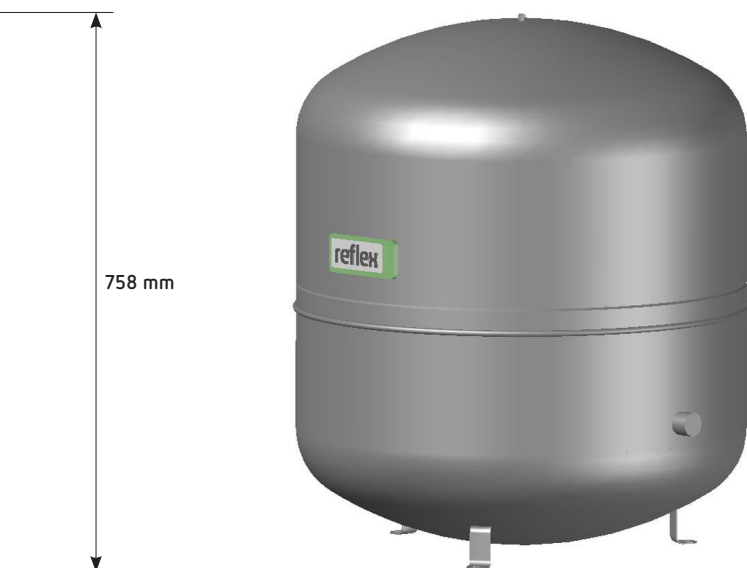
Reflex S 200 litri / 10 bar
