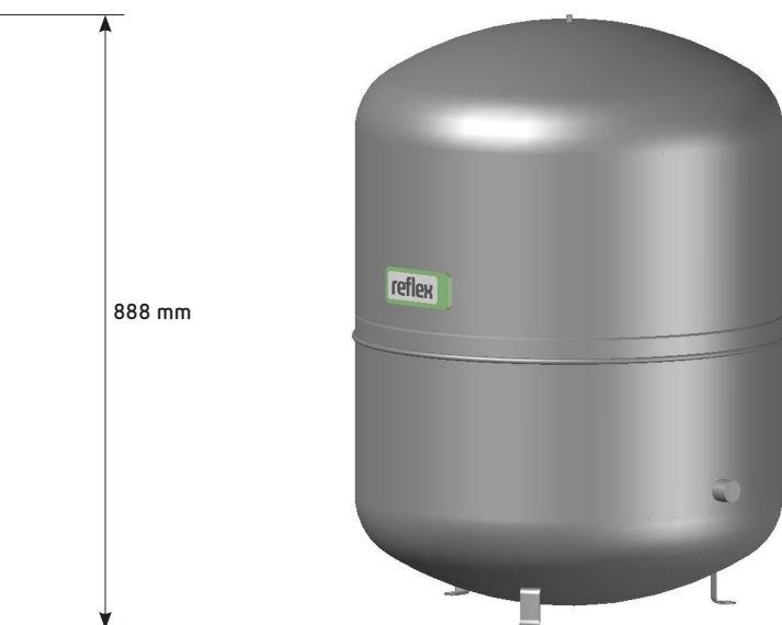
Reflex S 250 litri / 10 bar
