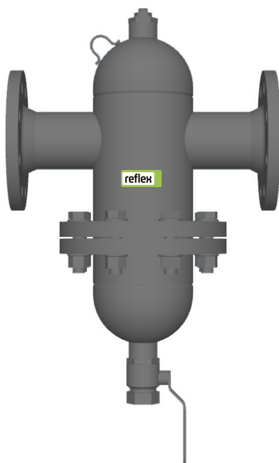
Exdirt D 65 R din oțel, cu flanșă de racord cu 4 găuri și flanșă de service
