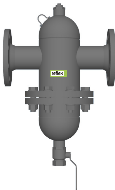
Exdirt D 65 R din oțel, cu flanșă de racord cu 8 găuri și flanșă de service
