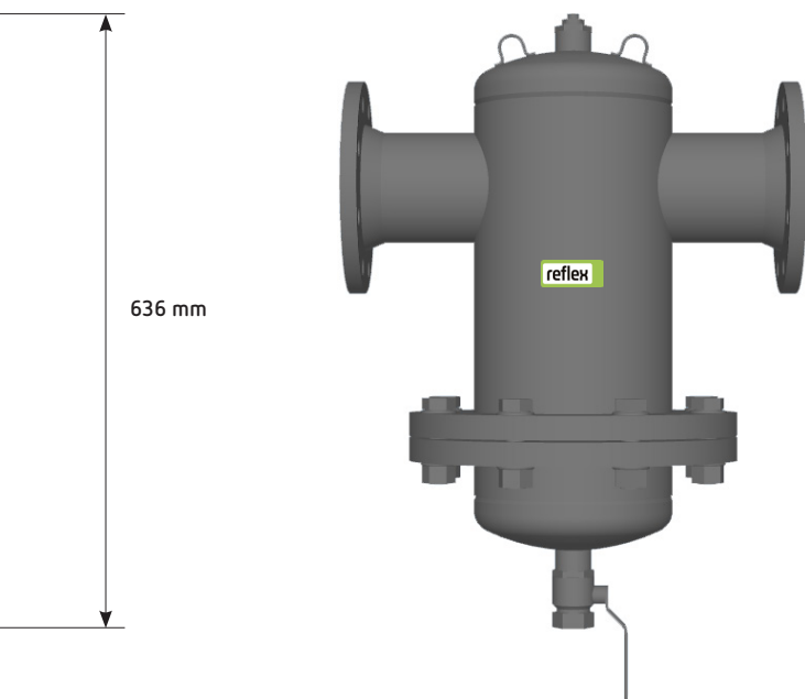
Exdirt D 100 R din oțel, cu flanșă de racord și flanșă de service
