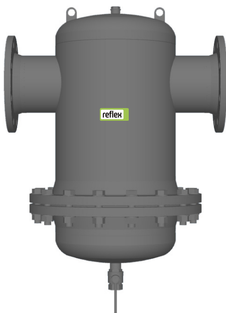
Exdirt D 150 R din oțel, cu flanșă de racord și flanșă de service
