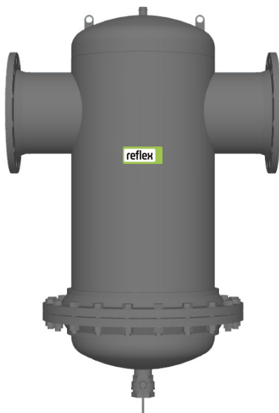
Exdirt D 250 R din oțel, cu flanșă de racord și flanșă de service
