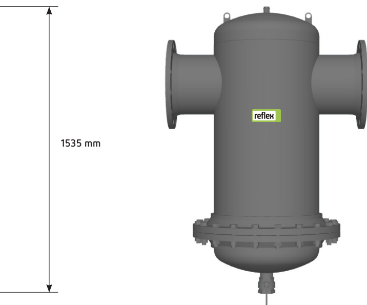
Exdirt D 300 R din oțel, cu flanșă de racord și flanșă de service
