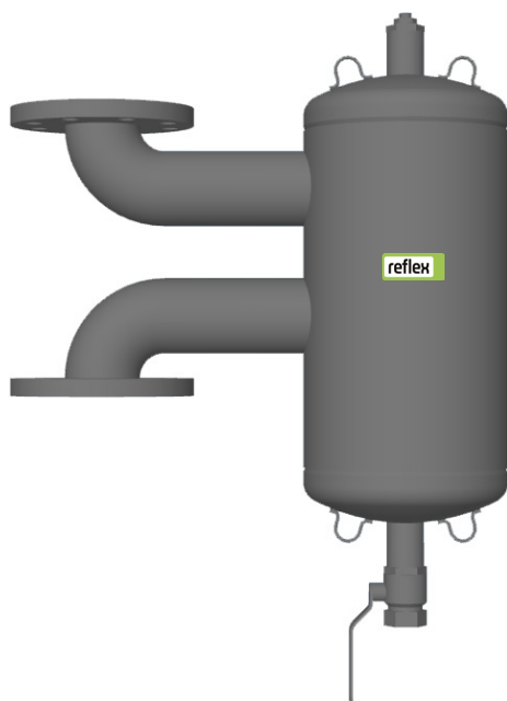
Exdirt D 65 V F1 din oțel, cu flanșă de racord, 10 bar
