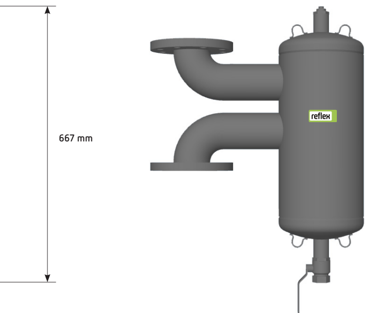
Exdirt D 80 V F1 din oțel, cu flanșă de racord, 10 bar
