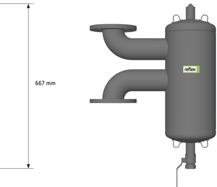
Exdirt D 80 V F1 din oțel, cu flanșă de racord, 6 bar
