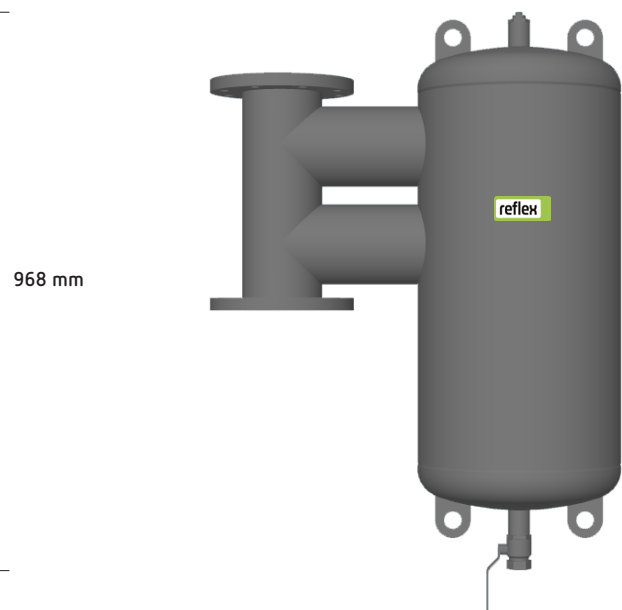
Exdirt D 125 V F1 din oțel, cu flanșă de racord, 10 bar
