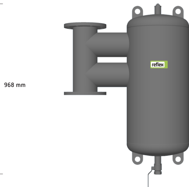
Exdirt D 125 V F1 din oțel, cu flanșă de racord, 6 bar
