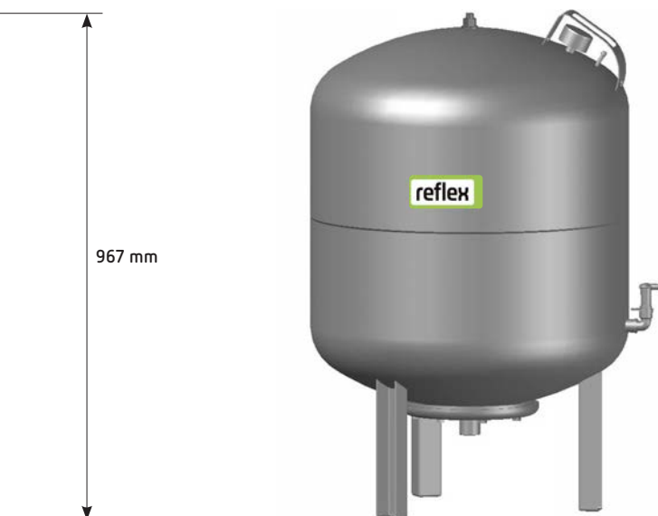
Reflex G 200 litri/6 bar
