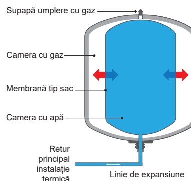
Schema funcțională vas de expansiune cu membrană tip sac (imagine cu caracter ilustrativ)
