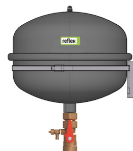
Ansamblu format din: vas de expansiune Reflex S 8-25 + cuplaj rapid SU 3/4x3/4 montat pe o consolă de perete cu colier de fixare. Componentele se comandă separat.
