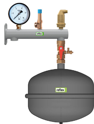
Ansamblu format din: vas de expansiune Reflex S 8-25 + cuplaj rapid SU 3/4x3/4 + ventil automat de aerisire + supapă de siguranță + manometru, montat pe o consolă de perete cu racorduri multiple. Componentele se comandă separat.
