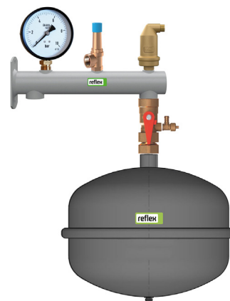
Ansamblu format din: vas de expansiune Reflex S 8-25 + cuplaj rapid SU ¾x¾ + ventil automat de aerisire + supapă de siguranță + manometru, montat pe o consolă de perete cu racorduri multiple. Componentele se comandă separat.
