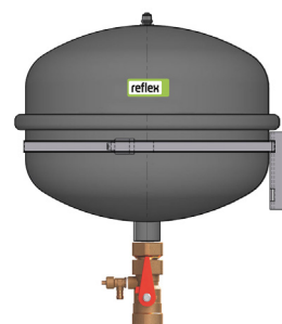
Ansamblu format din: vas de expansiune Reflex S 8-25 + cuplaj rapid SU ¾x¾ montat pe o consolă de perete cu colier de fixare. Componentele se comandă separat.
