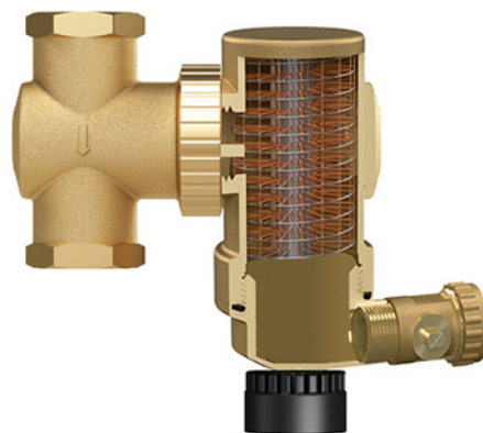
Această imagine este doar pentru ilustrarea aspectului interior al separatorului din alamă Exdirt Twist Magnet DT
