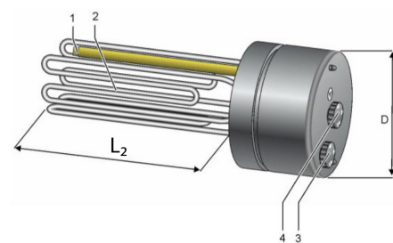
vedere isometrică EFHR 25.00
