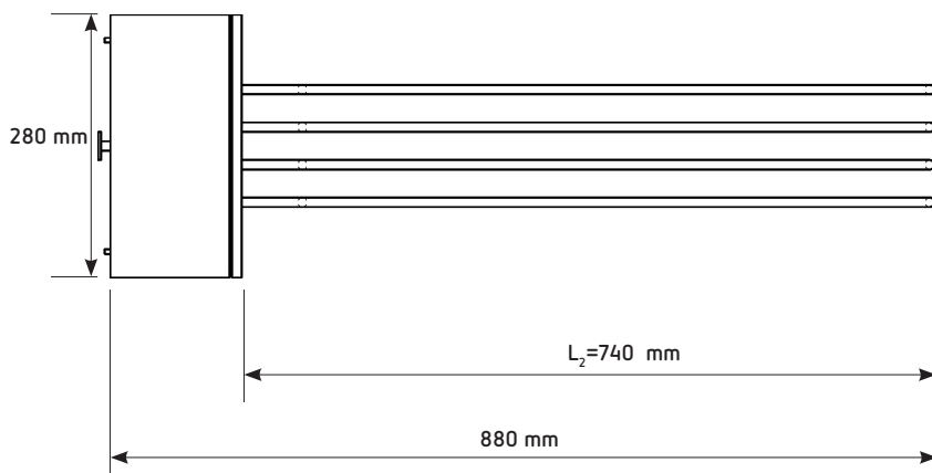
EFHR 25.00 – rezistență electrică, cu flanșă de montaj
