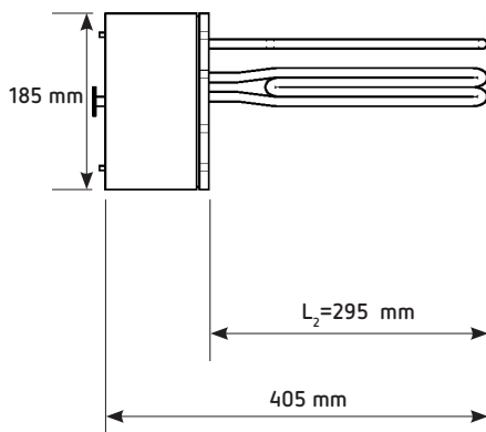
EFHR 4.00 – rezistență electrică, cu flanșă de montaj
