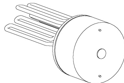
vedere isometrică EFHR 4.00
