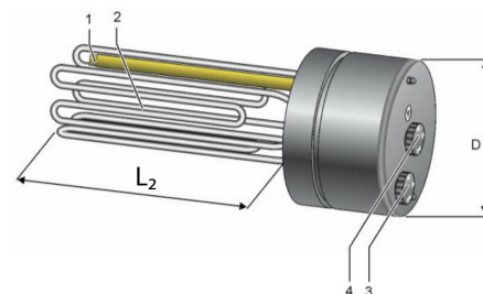
vedere isometrică EFHR 4.00
