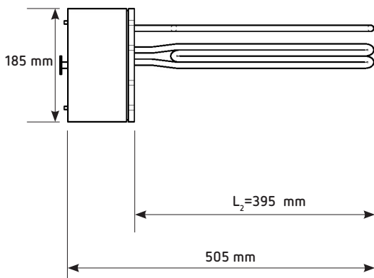
EFHR 6.00 – rezistență electrică, cu flanșă de montaj
