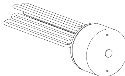
vedere isometrică EFHR 8.00
