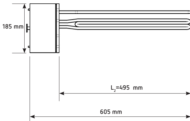
EFHR 8.00 – rezistență electrică, cu flanșă de montaj
