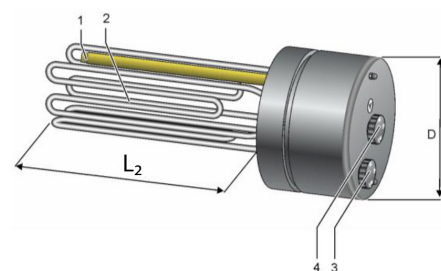
vedere isometrică EFHR 19.00
