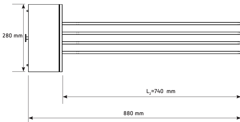
EFHR 19.00 – rezistență electrică, cu flanșă de montaj
