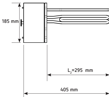
EFHR 2.50 – rezistență electrică, cu flanșă de montaj
