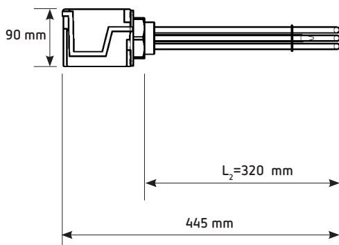
EEHR 2.00 – rezistență electrică, cu montaj prin înfiletare
