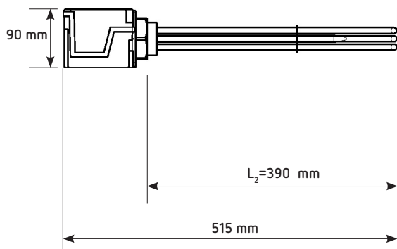
EEHR 3.00 – rezistență electrică, cu montaj prin înfiletare
