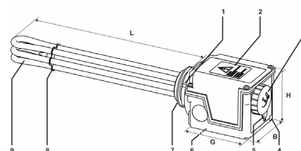
vedere isometrică EEHR 3.00
