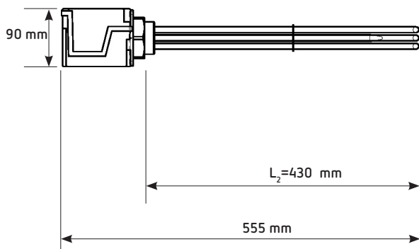
EEHR 3.80 – rezistență electrică, cu montaj prin înfiletare
