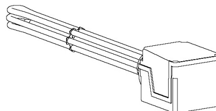
vedere isometrică EEHR 3.80
