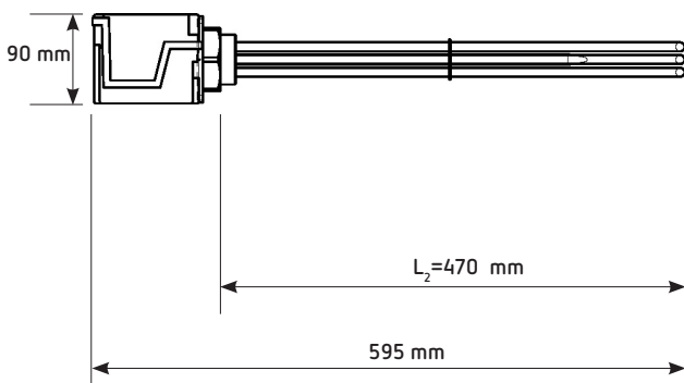
EEHR 4.50 – rezistență electrică, cu montaj prin înfiletare
