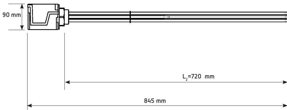
EEHR 7.50 – rezistență electrică, cu montaj prin înfiletare
