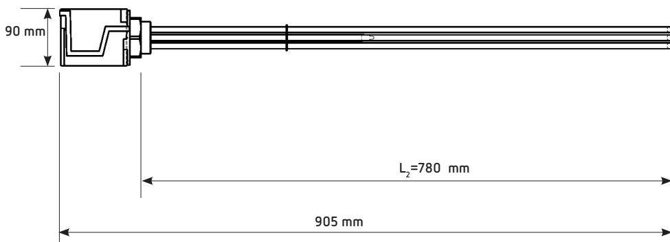
EEHR 9.00 – rezistență electrică, cu montaj prin înfiletare
