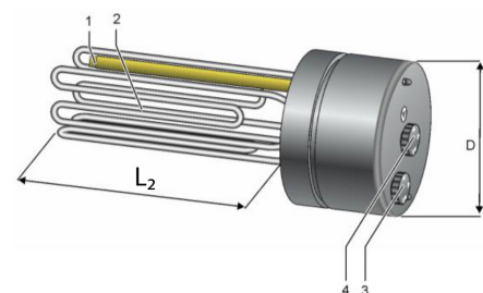
vedere isometrică EFHR 35.00
