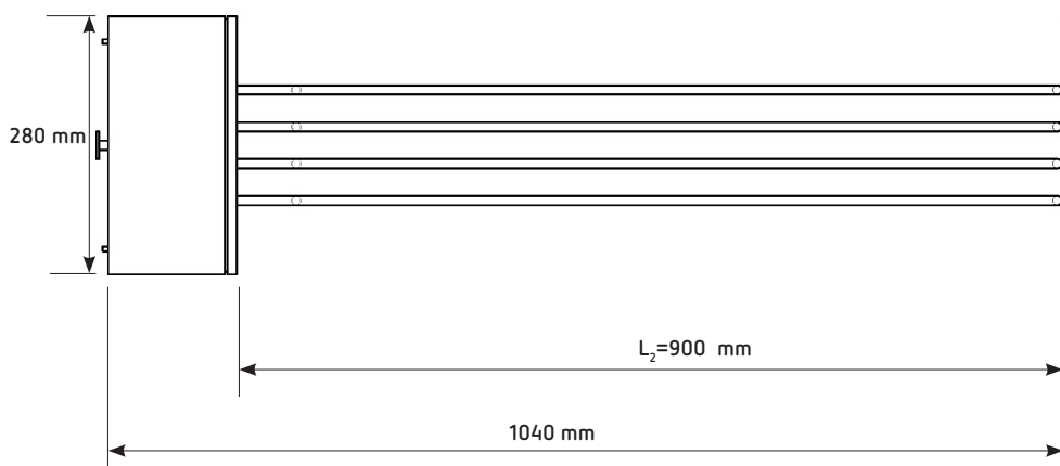
EFHR 35.00 – rezistență electrică, cu flanșă de montaj
